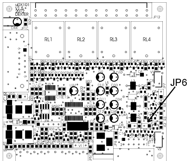
Placa impressa do \mu DX101
